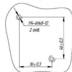
Место под усилитель согласующий ВК-312С-1
