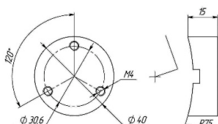
Магнит на трубу*
