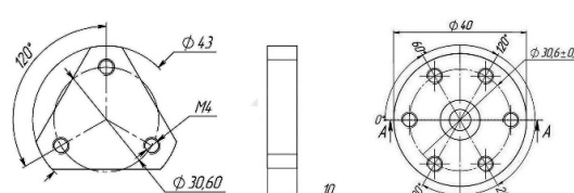
Магнит на плоскость*
