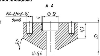
Конусная площадка
